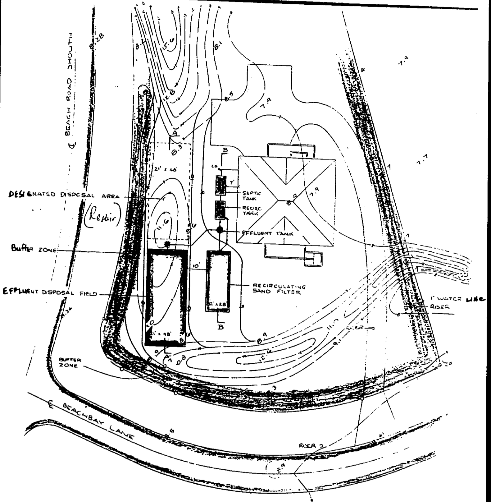
SITE PLAN - I BEACHBAY LANE
